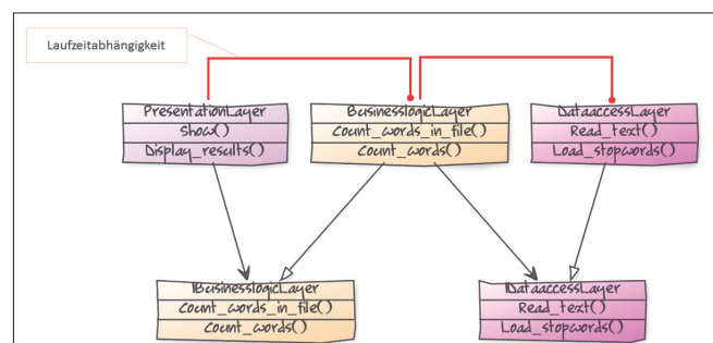
Mit DIP unterscheiden sich die Abhängigkeiten zur Compilezeit und zur Laufzeit (Bild 12)
